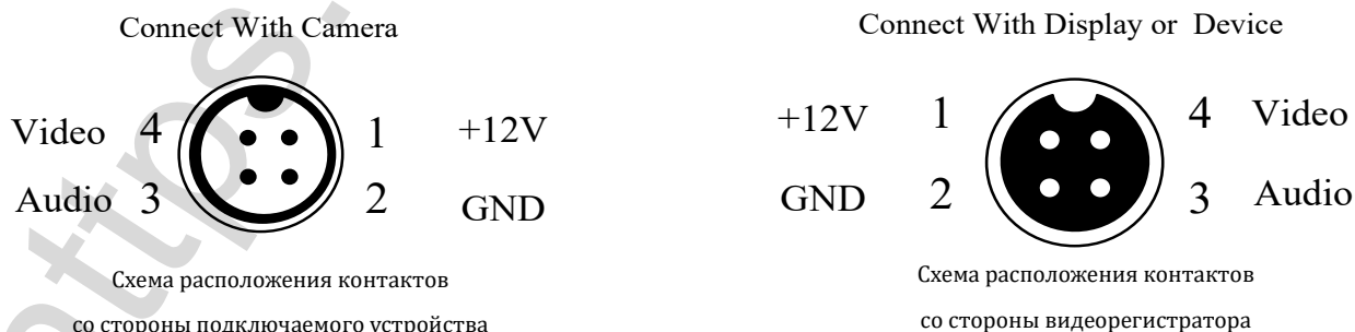
Рисунок 2.2 - Схемы расположения контактов со стороны подключаемого устройства и Видеорегистратора в разъемах типа GX
