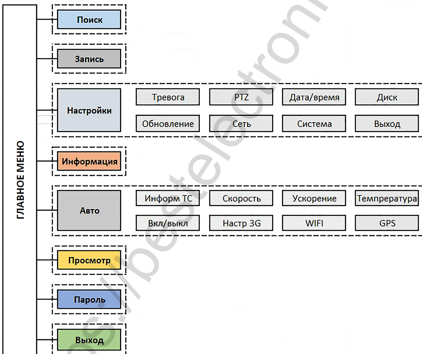
Рисунок 3.2 - Структура меню видеорегистратора MDR 8210 V1
