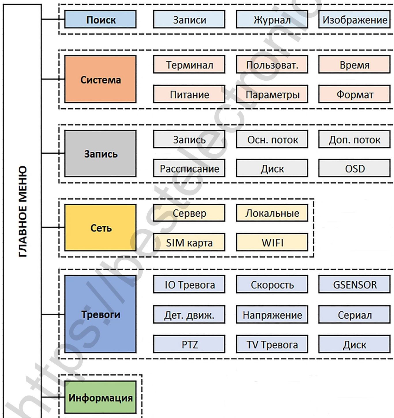
Рисунок 3.2 - Структура меню видеорегистратора MDR 8210 X
