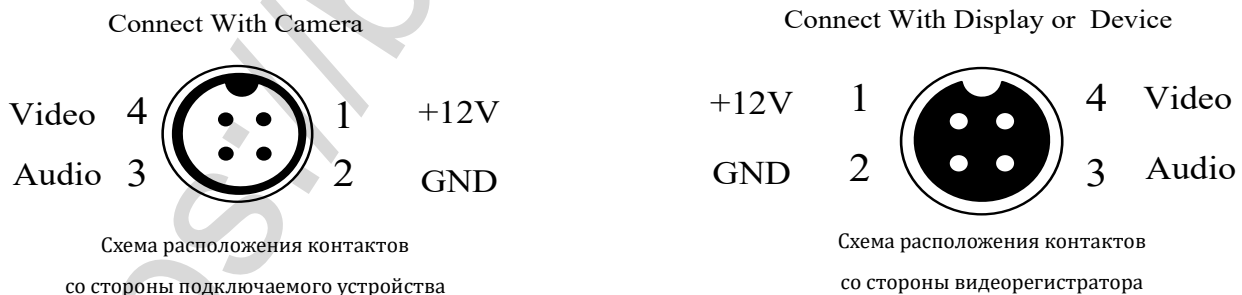
Рисунок 2.2 - Схемы расположения контактов со стороны подключаемого устройства и Видеорегистратора в разъемах типа GX
